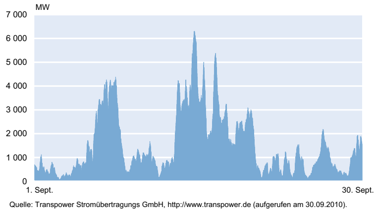
Abb. 1 Stromerzeugung aus Windkraftanlagen im Hochspannungsnetz von TENNET-Transpower im September 2010
