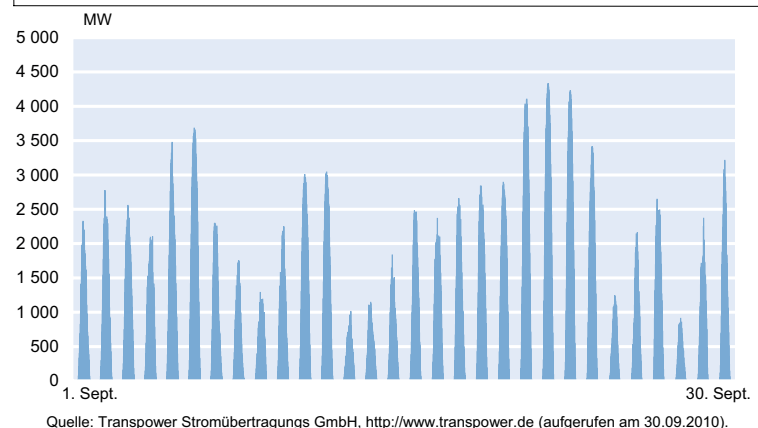
Abb. 2 Stromerzeugung aus Photovoltaikanlagen im Hochspannungsnetz von TENNET-Transpower im September 2010
